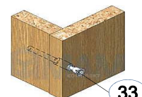
Евровинт 7 x 50
