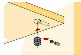
Рис.4 Схема установки эксцентрика
